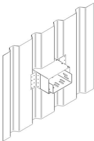
Prolaz za kabl kroz putanju
