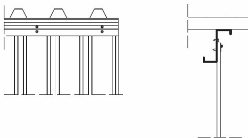
Primer instalacije čelične zavese mcr PROSMOKE ST duž grede
